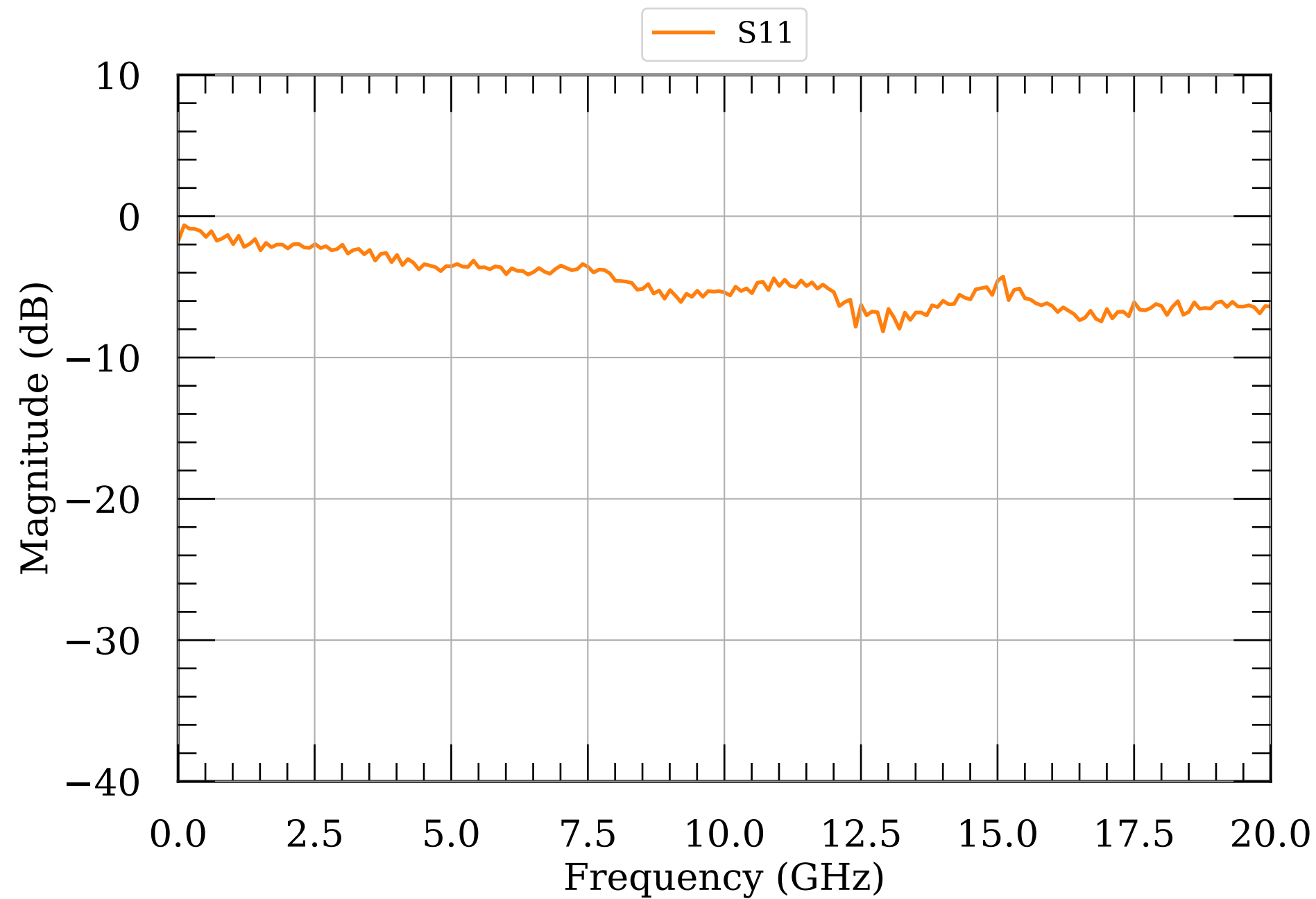
LNA S-params module022
